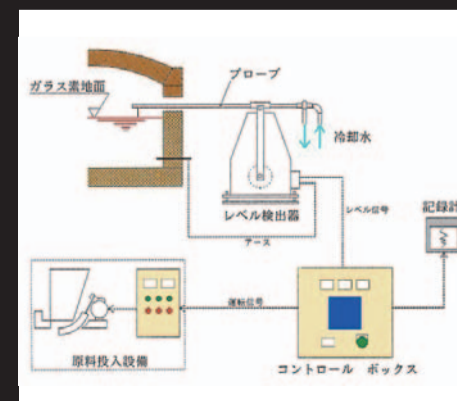
硝子レベラー概略図 Drawing of Glass Leveler
