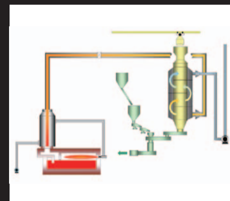
カレット予熱フロー Cullet Preheating System
