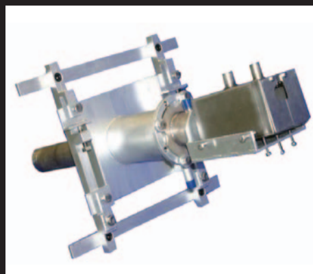
炉内監視カメラ ITV Camera
