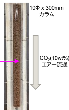
CO 2 固体回収材 (NaFeO 2 ペレット)
